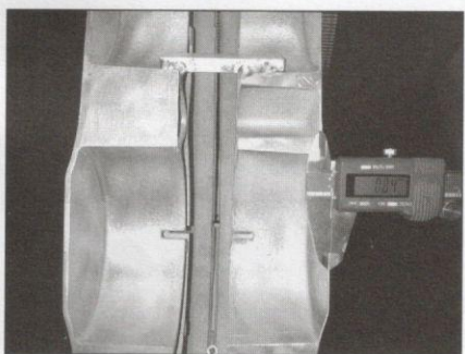
■ 4. kép. Vékony falú homoköntvény metszetei: a bal oldalon 540 mm hosszón 3 mm-es átlagos falvastagsággal, a jobb oldalon 540 mm hosszón 0,8-1,5 mm-es átlagos falvastagsággal
