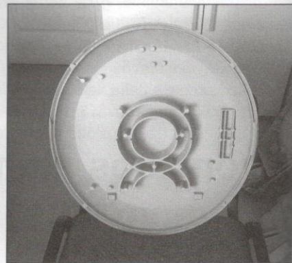
■ 6. kép. Vékony falú homokformázott öntvény 540 mm hosszón 3 mm-es átlagos falvastagsággal
