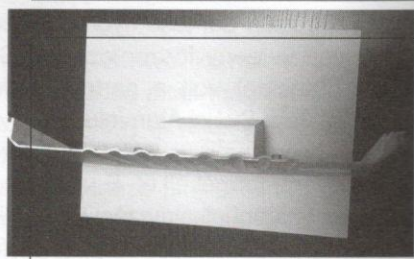
■ 7. kép. Vékony falú homokformázott öntvény 370 mm hosszón 2 mm-es átlagos falvastagsággal
