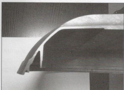
■ 3. kép. Vékony falú homokformázott öntvény 600 mm hosszón 2,7 mm-es átlagos falvastagsággal
