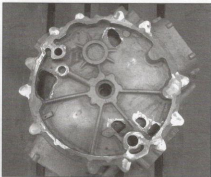
■ 1. kép. Nyersformában, maggal készült öntvény, 800 mm hosszón 10 mm-es átlagos falvastagsággal
